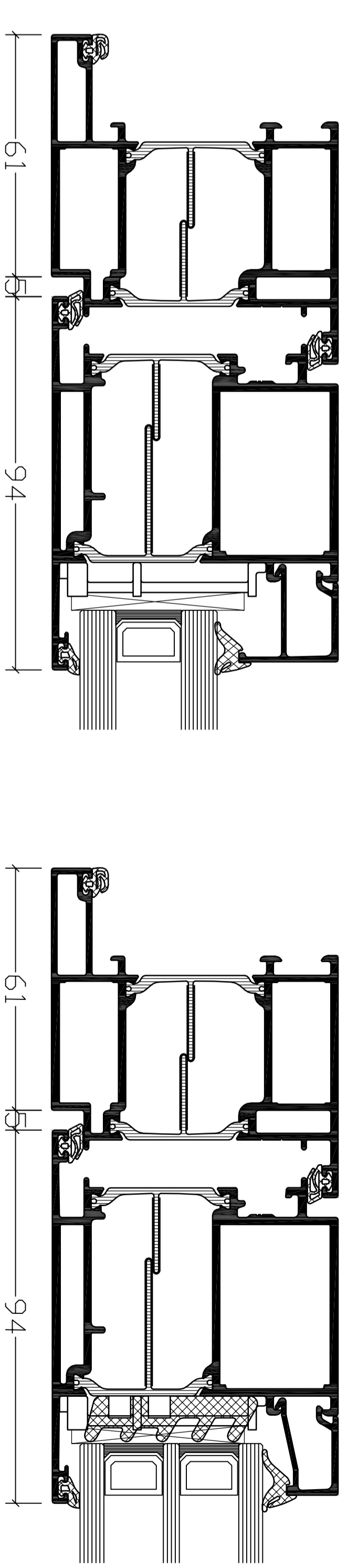
VARIATIES GLAS 1:1
