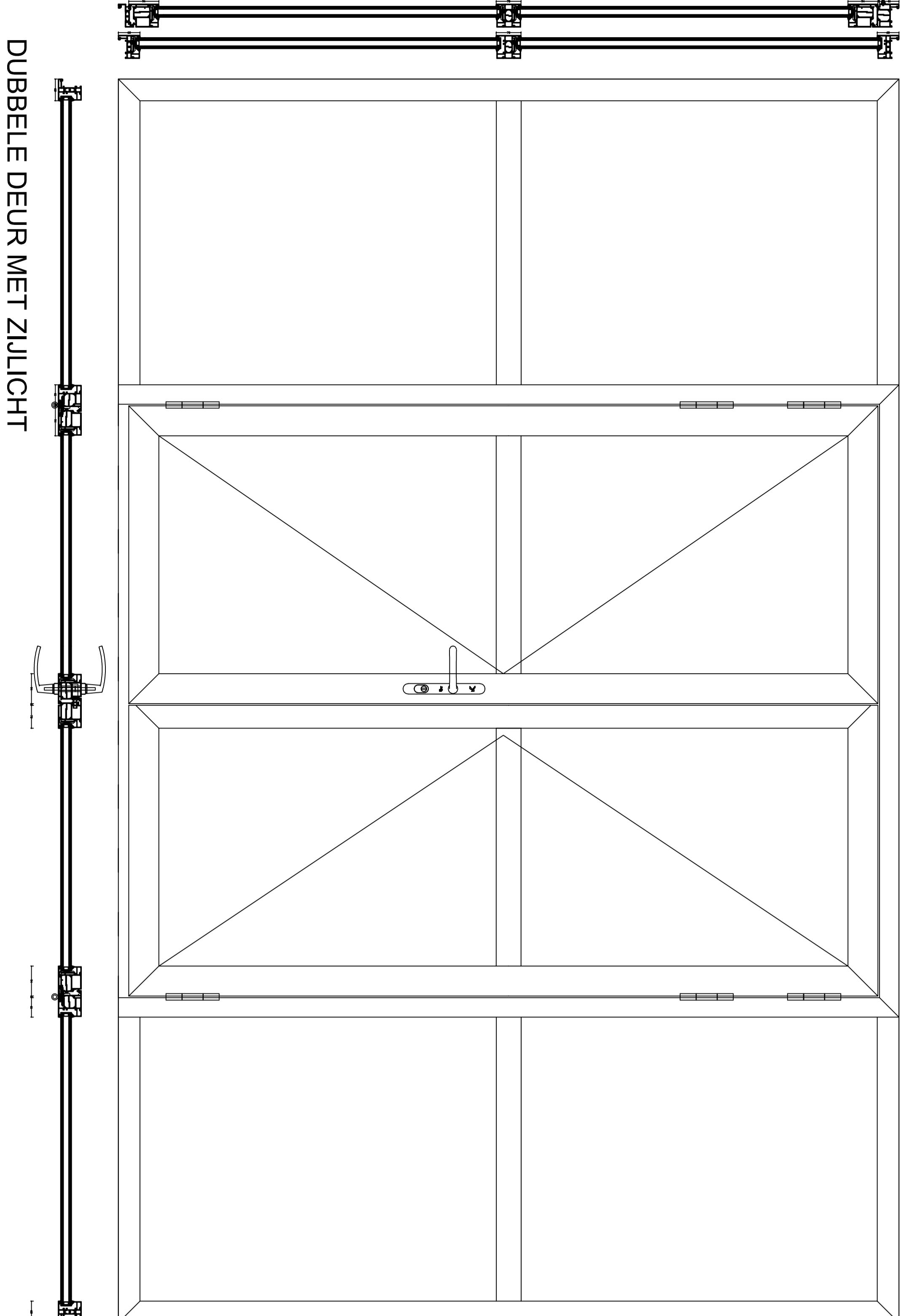
VARIATIES UITVOERING 1:2
