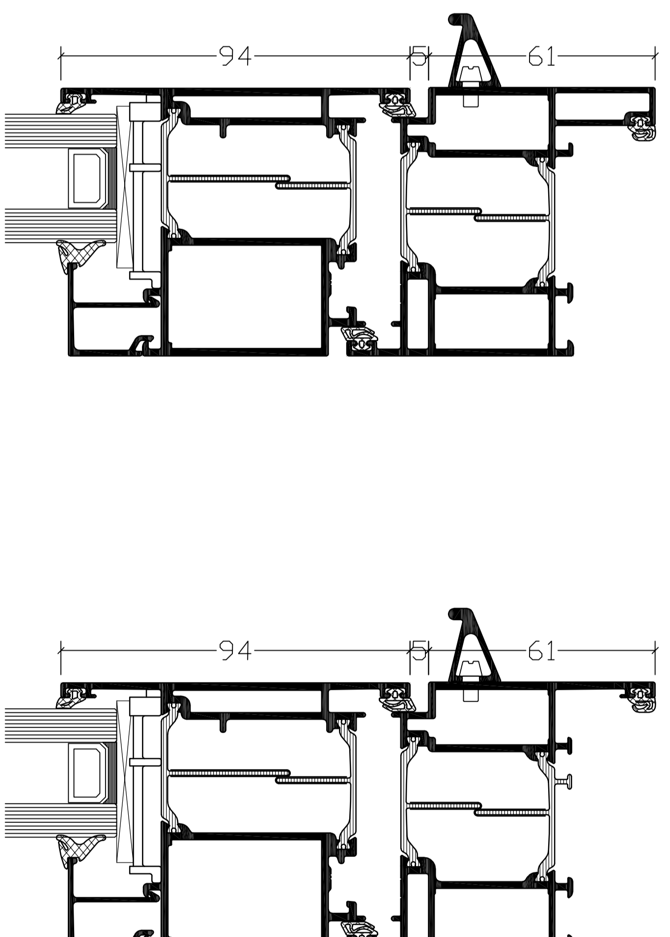
VARIATIES WATERAFVOER 1:1
